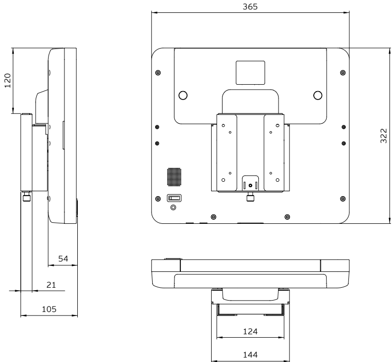
Abb. 6: POS Touch 15 inkl. Wandhalterung (Maße in Millimetern)
