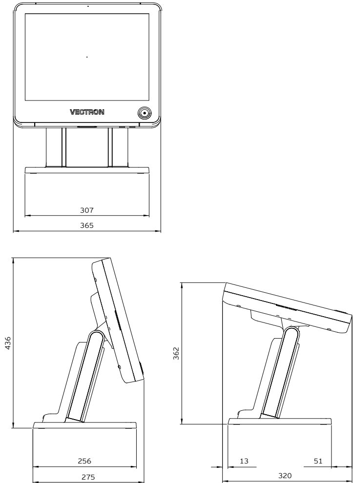
Abb. 4: POS Touch 15 inkl. Standfuß S420 (Maße in Millimetern)
