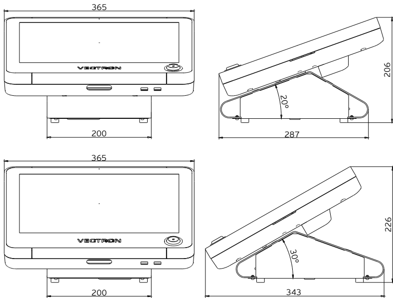
Abb. 5: POS Touch 15 inkl. Standfuß S500 (Maße in Millimetern)
