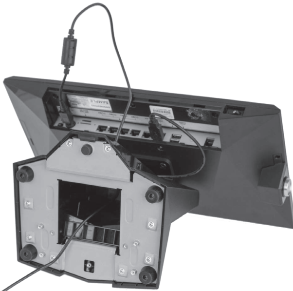
Abb. 7: Netzteil anschließen
