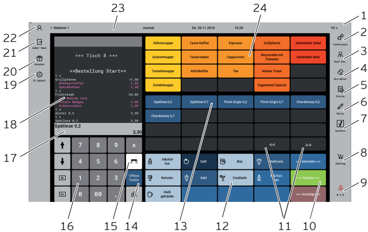
Abb. 10: Registrieroberfläche
