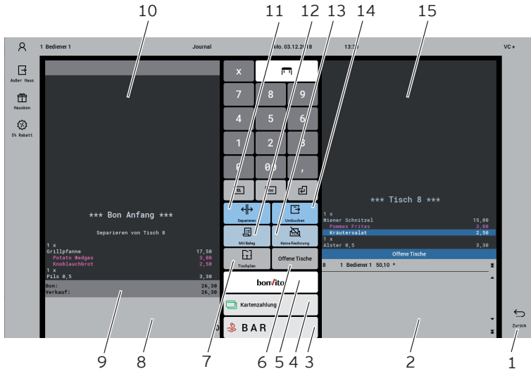
Abb. 11: Zahlungsoberfläche
